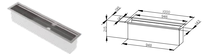
CANALE ATTREZZATO 3 MODULI VCA-3M Equipped track, 3 modules VCA-3M
