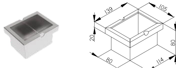
CONTENITORE PICCOLO CN105 Small container CN105
