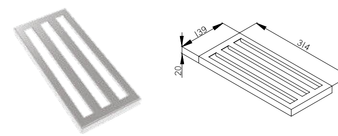
SUPPORTO TAGLIERE SPTG Chopping-board rack SPTG
