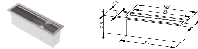
CANALE ATTREZZATO 2 MODULI VCA-2M Equipped track, 2 modules VCA-2M
