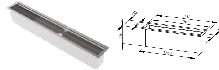
CANALE ATTREZZATO 4 MODULI VCA-4M Equipped track, 4 modules VCA-4M
